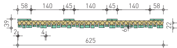
Längsschnitt:
