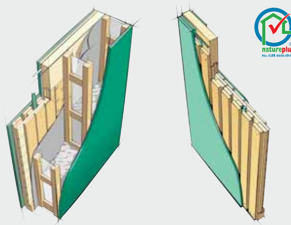
Aussenwand hoch wärmegeklämt
